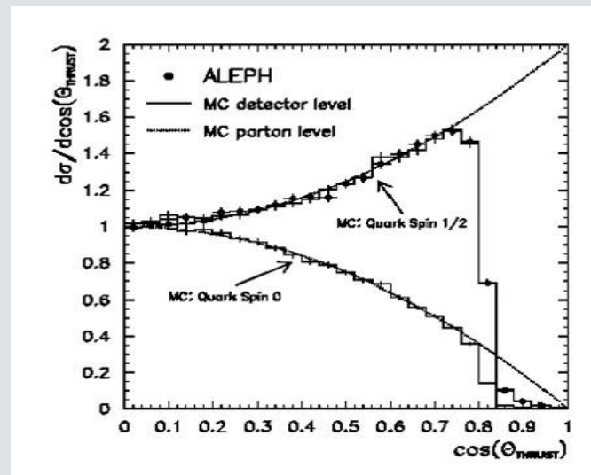
ALEPH (LEP) E = 90 \text{ GeV}
