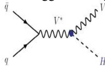
Higgsstrahlung
