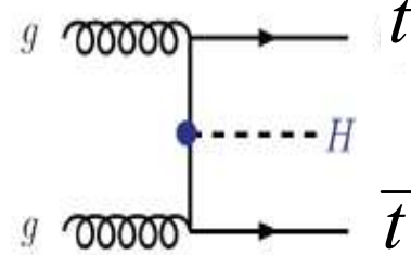
Ht\bar{t}
